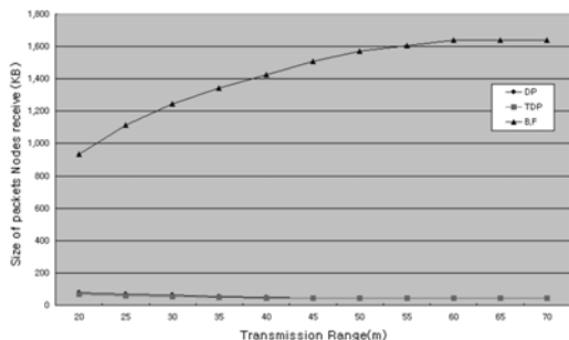
그림 9 노드가 80인 네트워크에서 노드가 수신한 패킷의 크기
