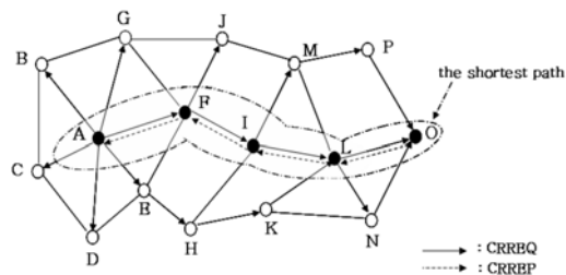
그림 5 CRREP 패킷의 전송
