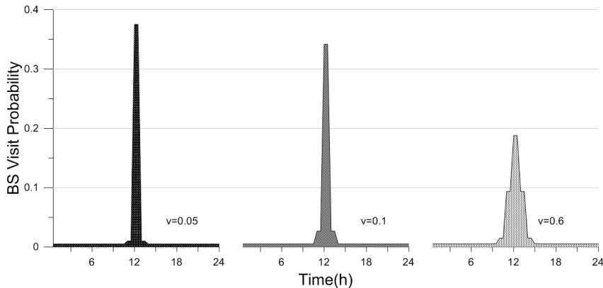
그림 2. 분산 v 에 따른 BS의 방문 확률 p_{\text{slot}} (30분 기준) Fig. 2. BS visiting probability p_{\text{slot}} by variant v (in 30 minutes)
