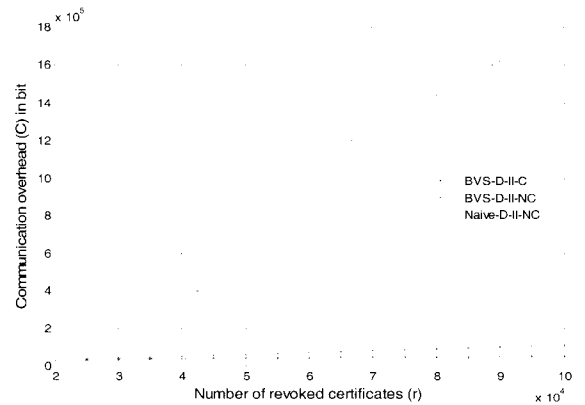
(그림 7) BVS-D-II-C와 Naive-D-II-C의 통신 오버헤드
