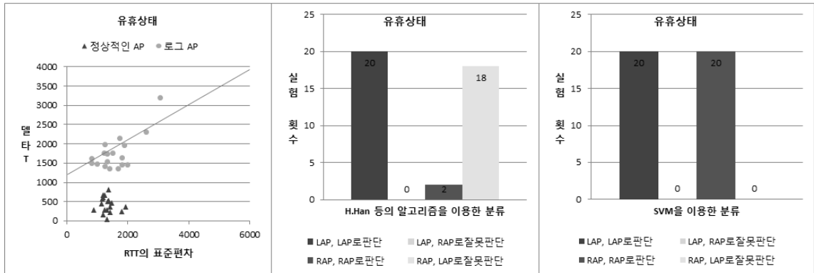
(그림 9) 채널 유휴상태일 때의 로그 AP와 정상적인 AP의 데이터 분포도와 H.Han등의 알고리즘을 적용한 로그 AP 탐지결과와 SVM을 이용한 로그 AP 탐지 결과
