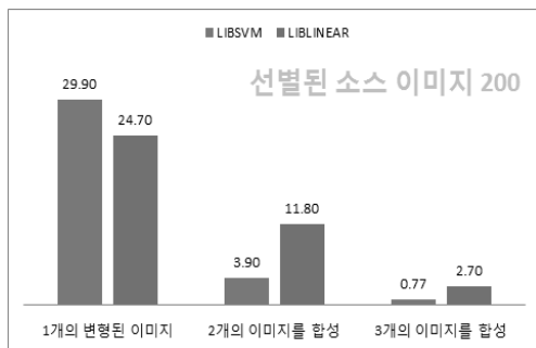
[그림 4] 200개의 소스 이미지를 선별한 경우의 시나리오 1의 실험 결과 (단위: %)
