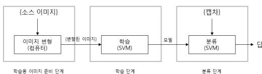
(그림 2) 시나리오 1의 실험 방법
