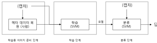
(그림 6) 시나리오 2의 실험 방법
