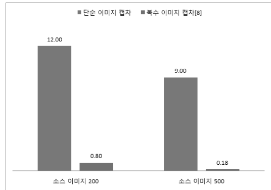
(그림 7) 시나리오 2에서의 단순 이미지 캡처와 복수 이미지 캡처의 비교 결과(LIBSVM, 단위: %)
