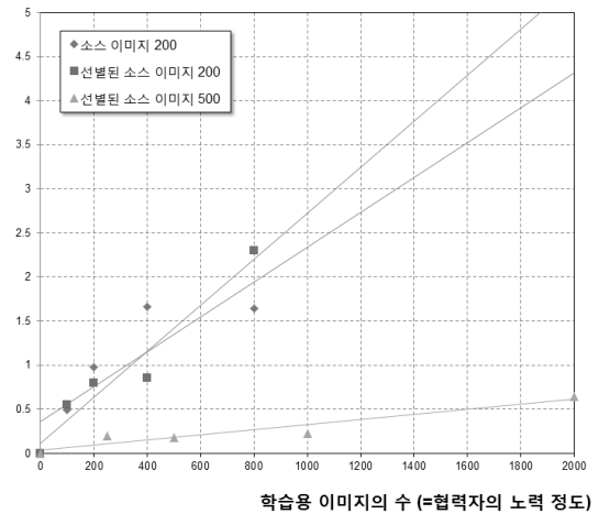
(그림 8) 시나리오 2에서의 협력자의 노력에 따른 성공 확률 비교 (테스트 이미지는 각각 1000개, LIBSVM [24] 사용) (단위: %)
