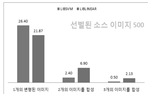
[그림 5] 500개의 소스 이미지를 선별한 경우의 시나리오 1의 실험 결과 (단위: %)
