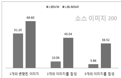
[그림 3] 200개의 소스 이미지를 선별하지 않은 경우의 시나리오 1의 실험 결과
