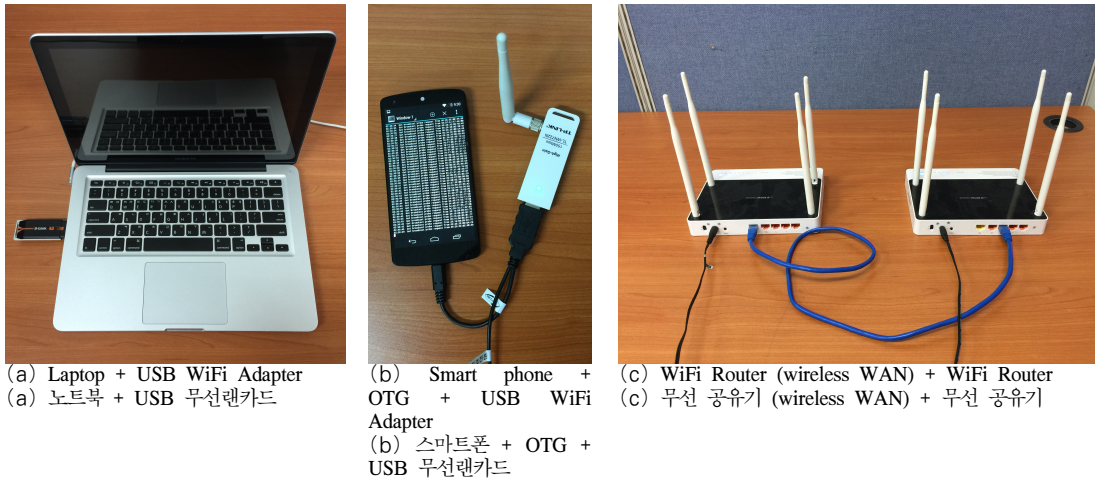
그림 1. 비인증 AP를 구성하는 다양한 방법들 Fig. 1. Various methods of configuring unauthorized APs
