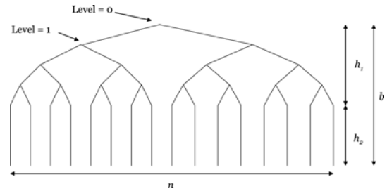
그림 3. 이진 탐색 트리의 작동 모델[1] ( h1 :완전 이진트리가 구성되는 부분, h2 :완전 이진트리가 구성되지 않는 부분, n : 태그의 개수, b : 태그의 비트수)
