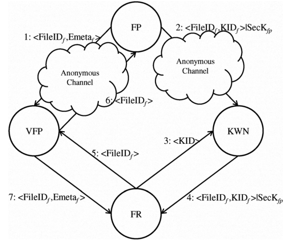
Fig. 1. A-Kad model
