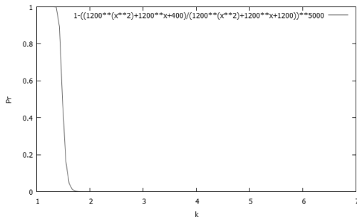
(그림 1) k 값 변화에 따른 시물레이션 실패확률
