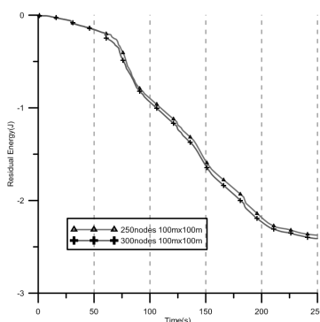
[그림 11] 센서 노드 밀도를 그리드 당 2.5개, 3개로 설정한 경우
