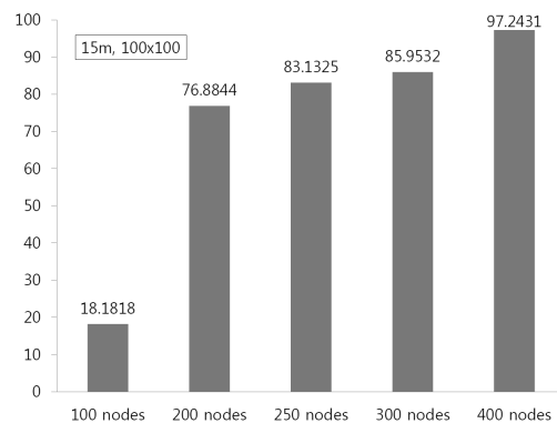
(그림 14) 노드 밀도에 따른 가용율 변화
