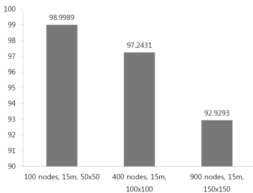
(그림 13) 노드의 개수에 따른 가용율 변화
