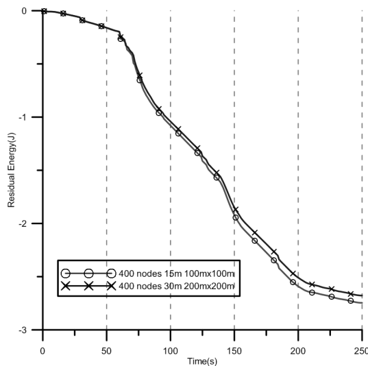
[그림 5] 400개의 센서 노드에서 통신 반경을 15m, 30m으로 하였을 경우
