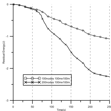
[그림 10] 센서 노드 밀도를 그리드 당 1개, 2개로 설정한 경우
