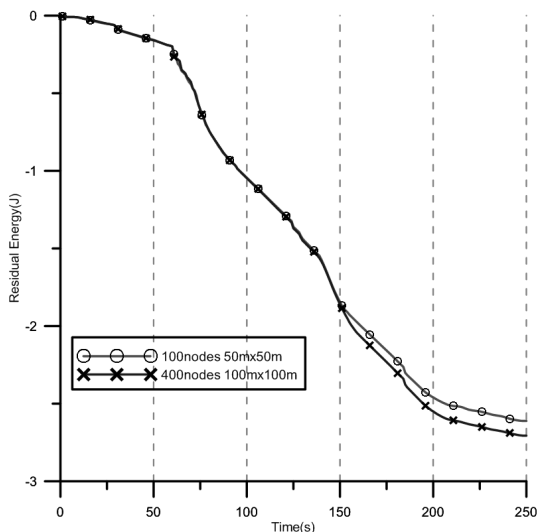
[그림 8] 센서 노드의 수를 각각 100개, 400개로 하였을 경우
