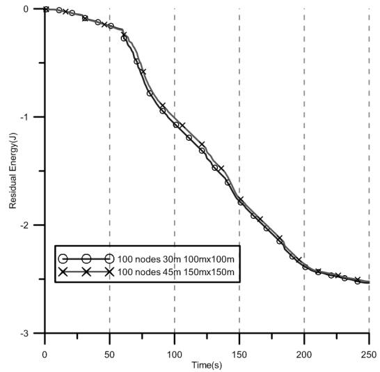
[그림 4] 100개의 센서 노드에서 통신 반경을 30m, 45m으로 하였을 경우
