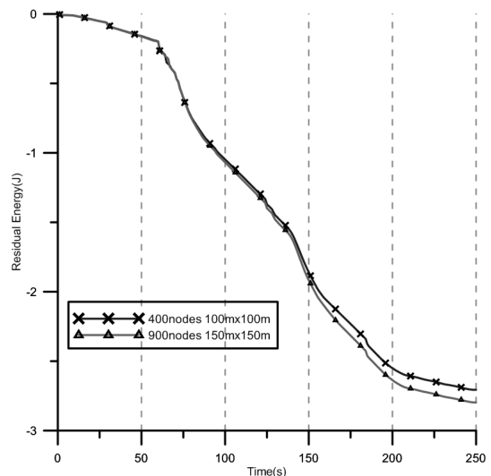
[그림 9] 센서 노드의 수를 각각 400개, 900개로 하였을 경우
