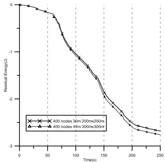
[그림 6] 400개의 센서 노드에서 통신 반경을 30m, 45m으로 하였을 경우
