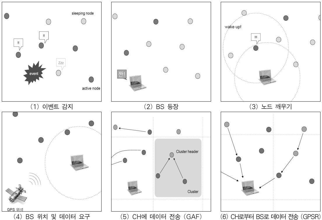
[그림 2] 모의실험을 위한 시나리오 주요 구성
