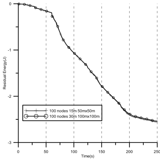
[그림 3] 100개의 센서 노드에서 통신 반경을 15m, 30m으로 하였을 경우
