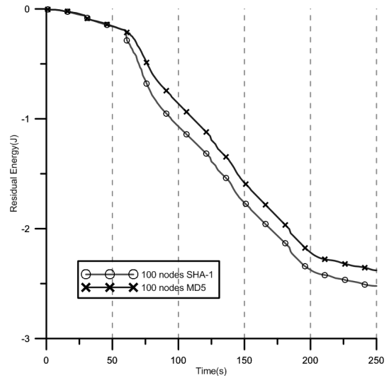
[그림 7] 사용되는 해시 함수를 SHA-1과 MD5로 하였을 경우
