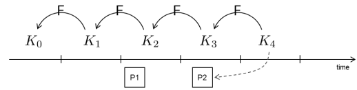
(그림 1) 키 체인을 이용한 \mu TESLA의 구현
