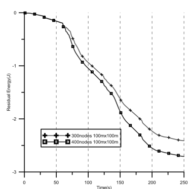
[그림 12] 센서 노드 밀도를 그리드 당 3개, 4개로 설정한 경우
