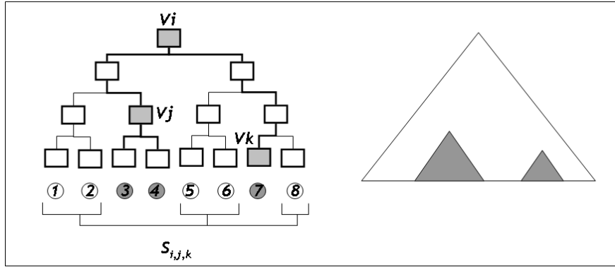
그림 1. 2-Subset Difference scheme에서의 부분집합 S_{i,j,k}
